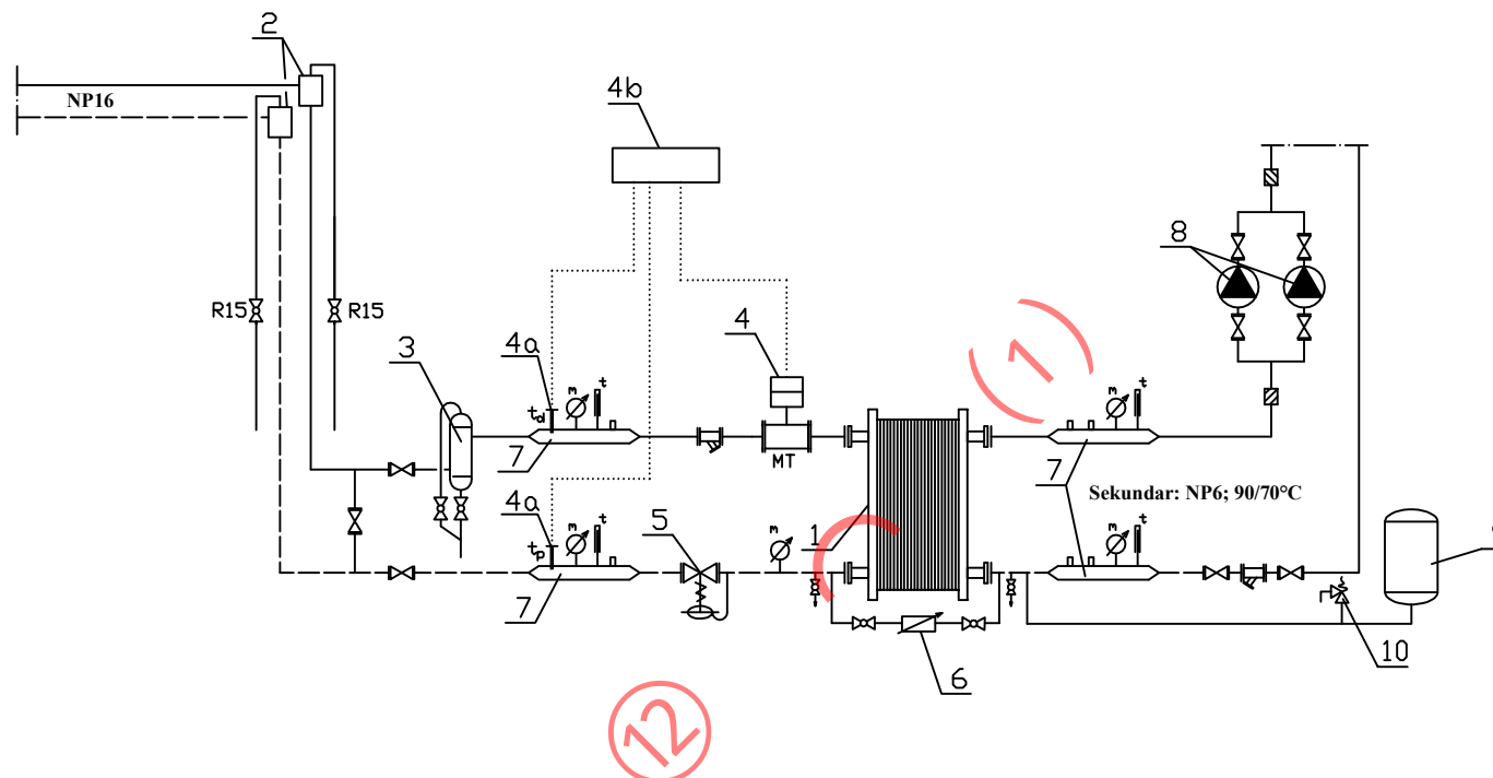
Цртеж 05: Типска топлотна подстанција капацитета мањег или једнаког 50KW, са затвореним експанзионим судом са мембрано
