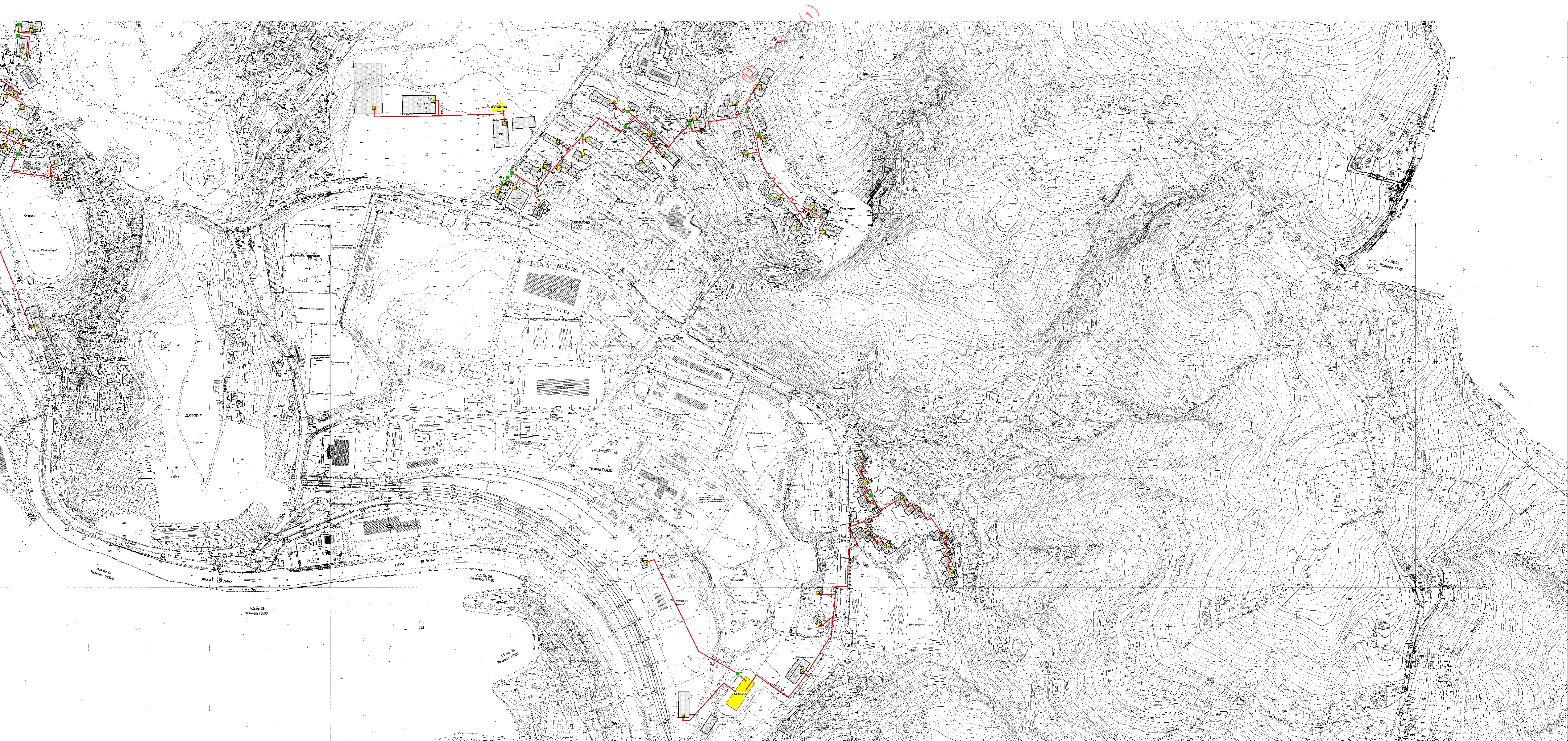
Цртеж 02: Насеље Крчагово- локације котларница и топловодна мрежа
